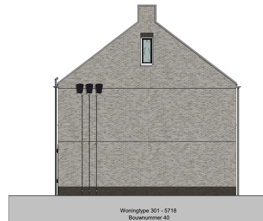
Rechtergevel Nestkasten en spandraden zijn indicatief ingetekend
